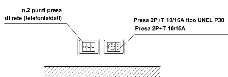
PARTICOLARE POSTAZIONE DI LAVORO
